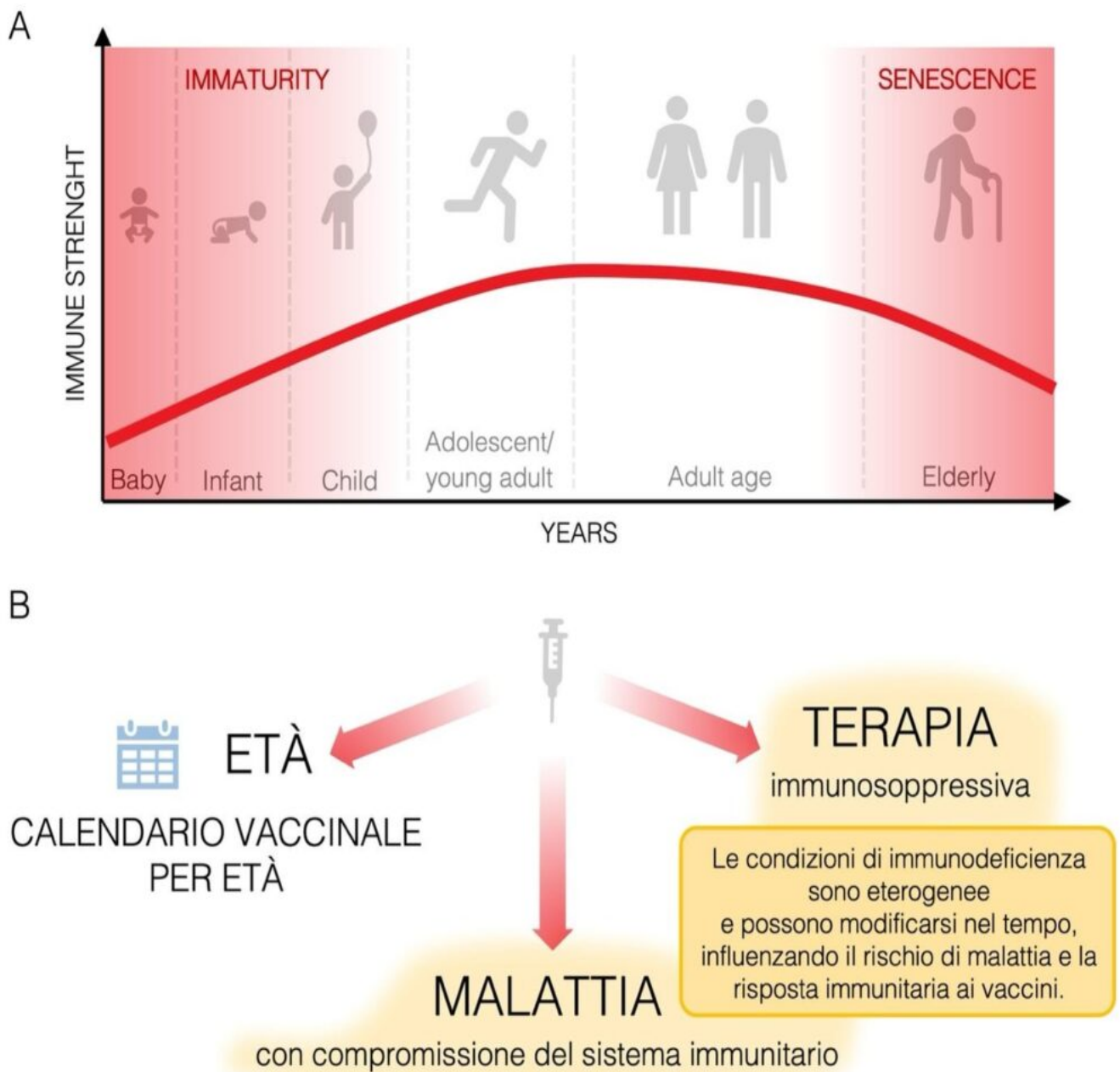
Figura 1. Le tre variabili della fragilità immunitaria ( immune frailty ). La fragilità del sistema immunitario è determinata dall'interazione di tre fattori principali: età, malattie e terapie. La sovrapposizione dei tre cerchi rappresenta l'aumento del grado di fragilità immunitaria quando più fattori coesistono nello stesso individuo.
